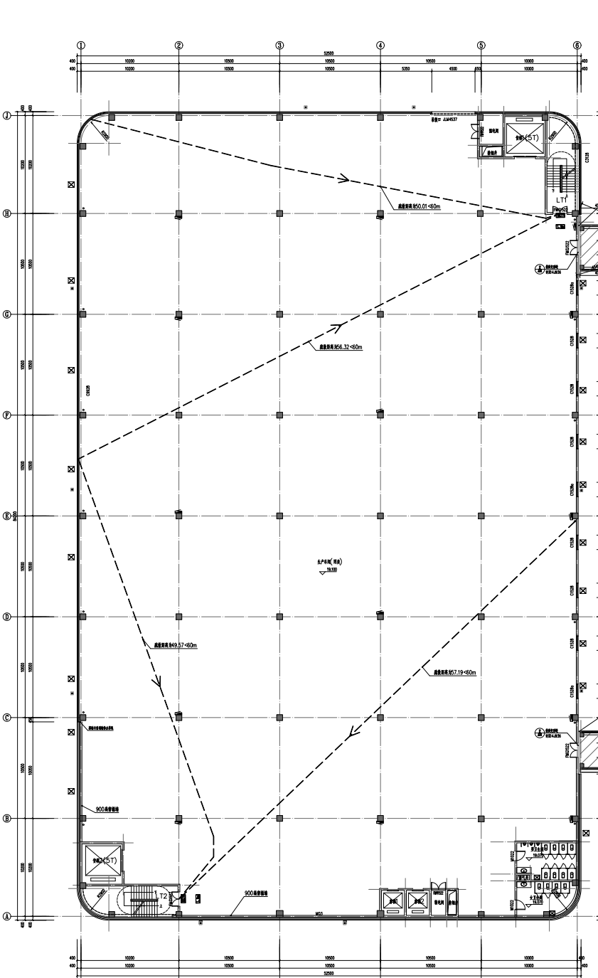
3#生产厂房 四层平面图
