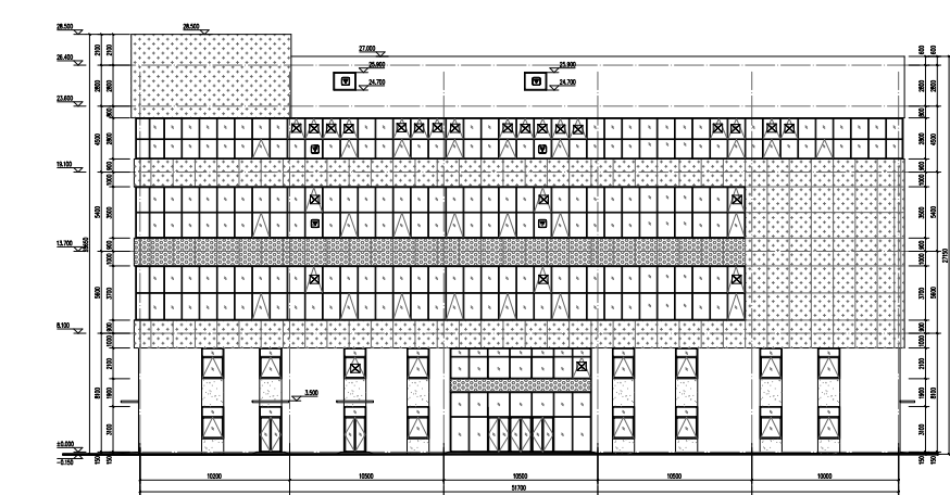
3#生产厂房 ①-⑥立面图
