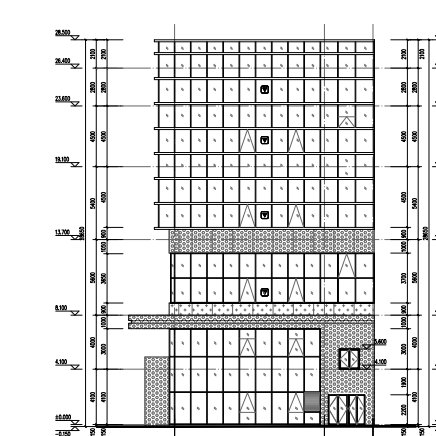
1#办公楼 ④-⑥立面图
