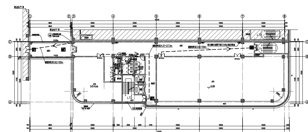
1#办公楼 四层平面图
