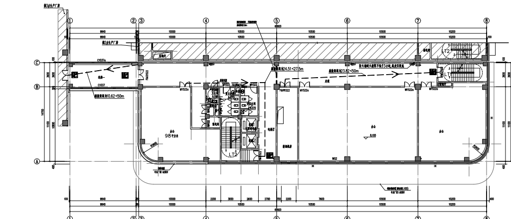
1#办公楼 三层平面图
