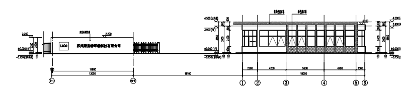
4#门卫 ①-⑥立面图
