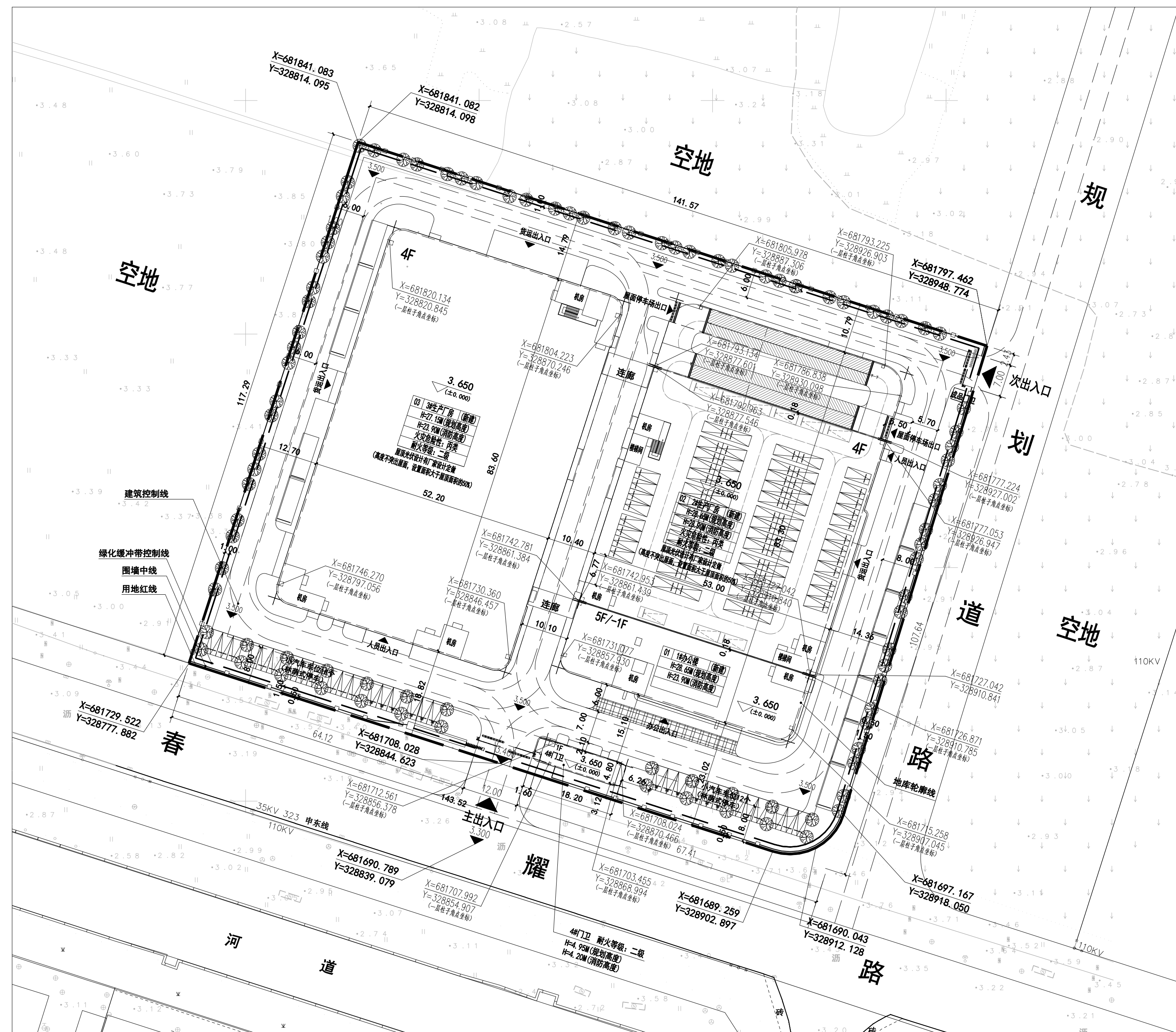
总平面图
