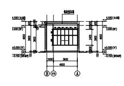
4#门卫 B-A立面图
