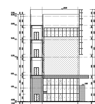
1#办公楼 ③-①立面图
