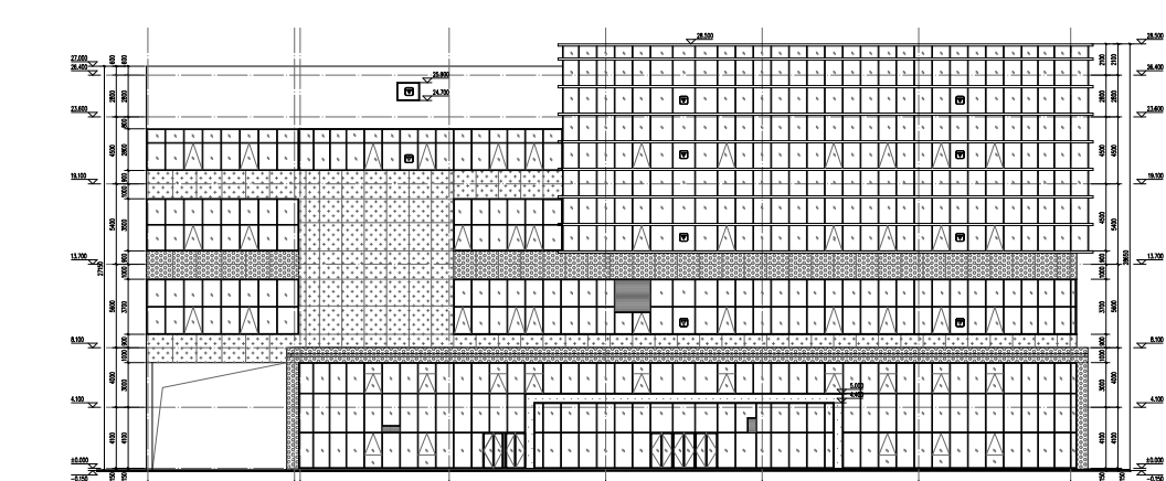
1#办公楼 ①-⑧立面图
