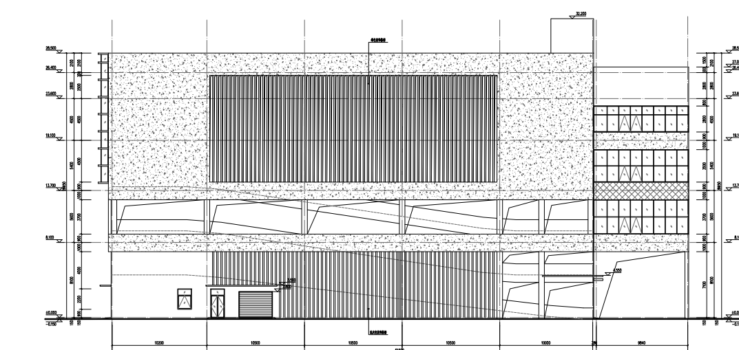
2#生产厂房 8-1立面图
