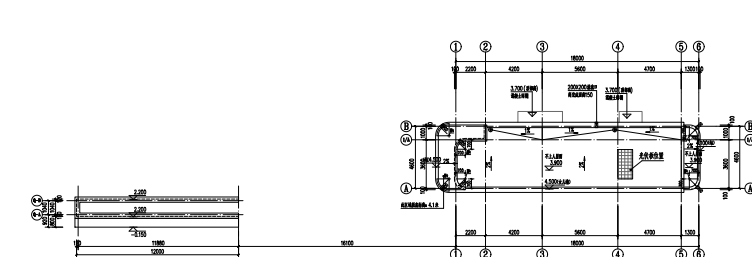
4#门卫 屋顶层平面图
