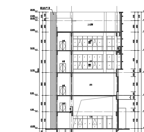
1#办公楼 1-1剖面图
