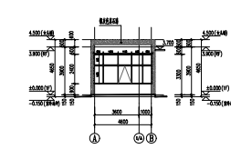
4#门卫 A-B立面图
