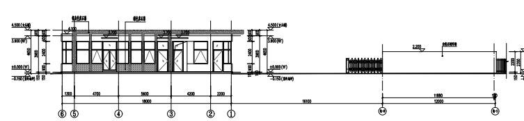
4#门卫 ⑥-①立面图
