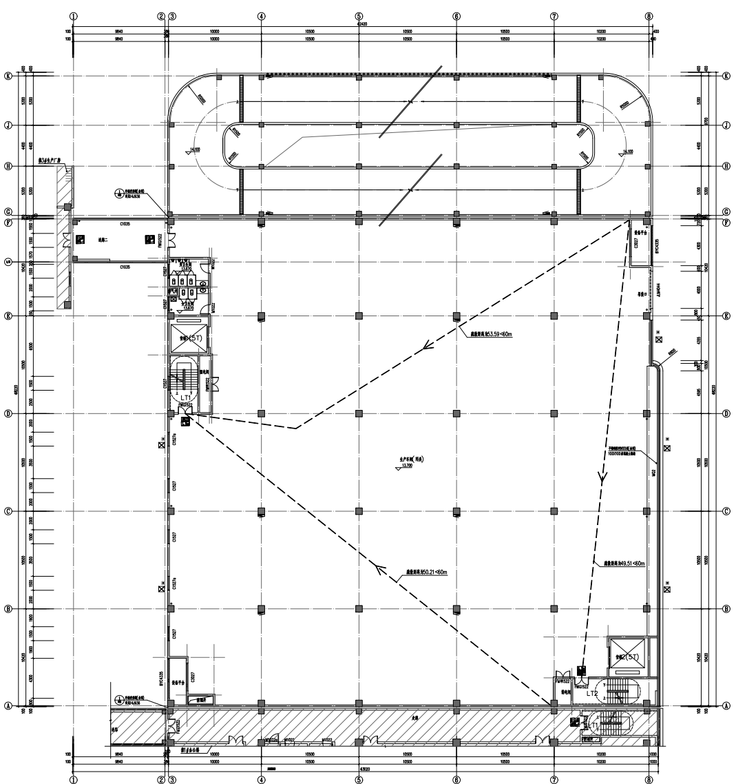
2#生产厂房 三层平面图
