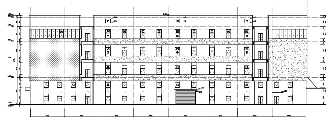
3#生产厂房 A-J立面图
