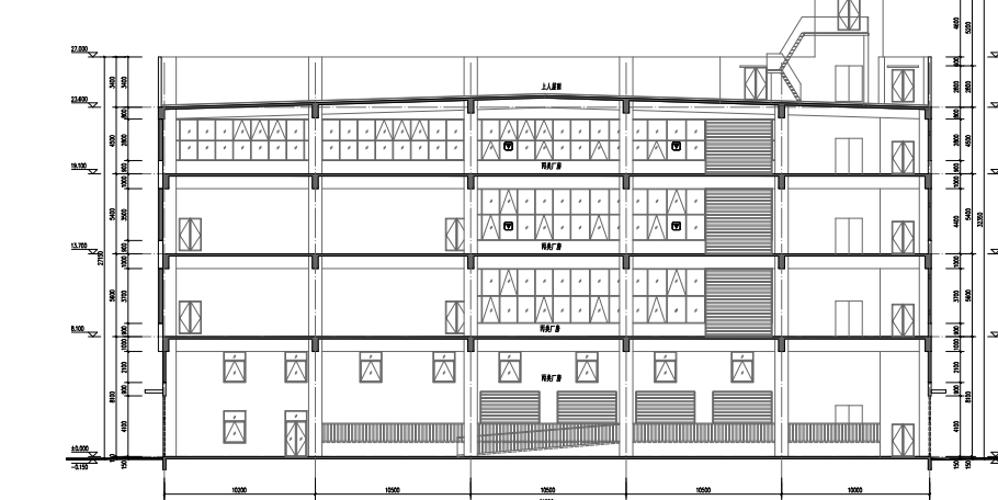
3#生产厂房 1-1剖面图
