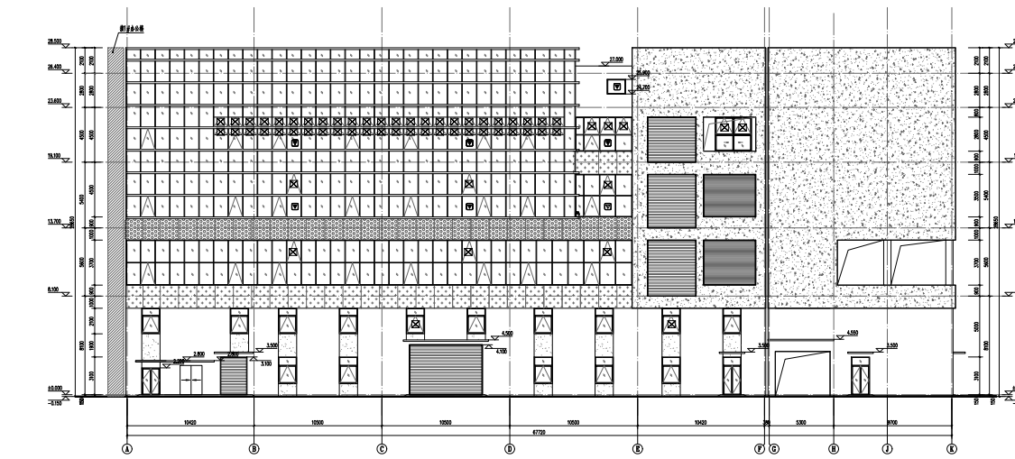
2#生产厂房 A-K立面图
