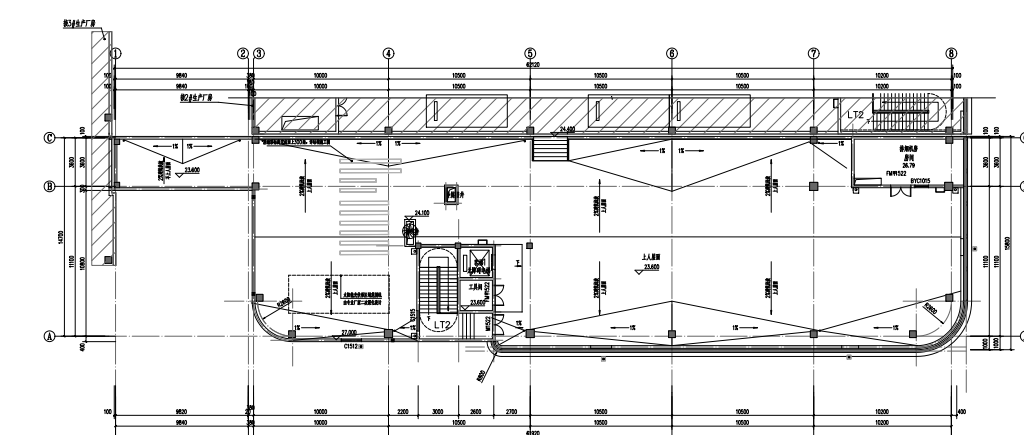
1#办公楼 机房层平面图
