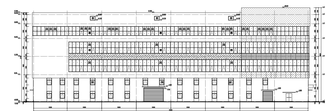
3#生产厂房 J-A立面图
