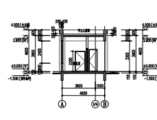
4#门卫 1-1剖面图
