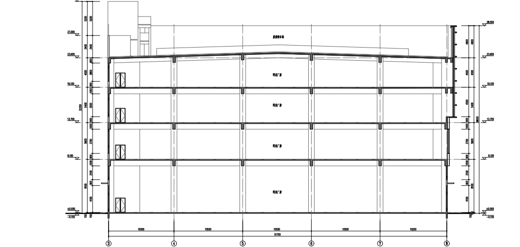
2#生产厂房 1-1剖面图
