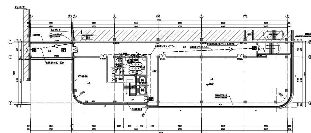
1#办公楼 五层平面图
