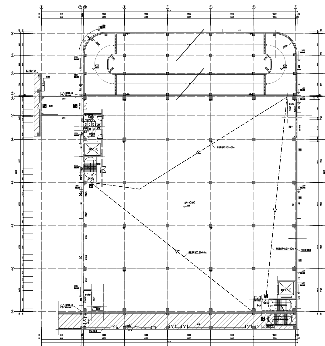
2#生产厂房 二层平面图
