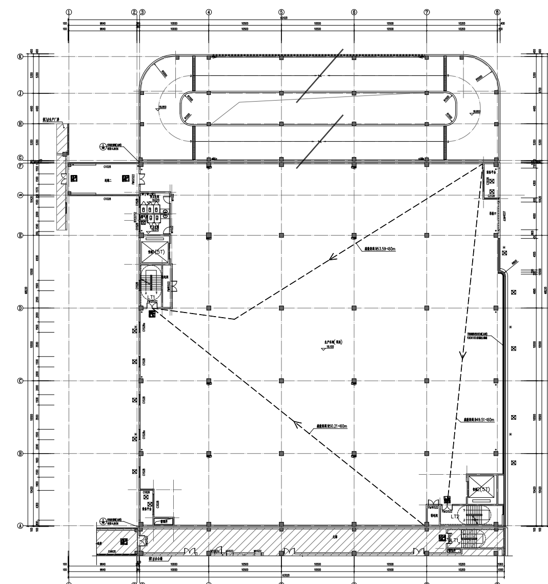
2#生产厂房 四层平面图
